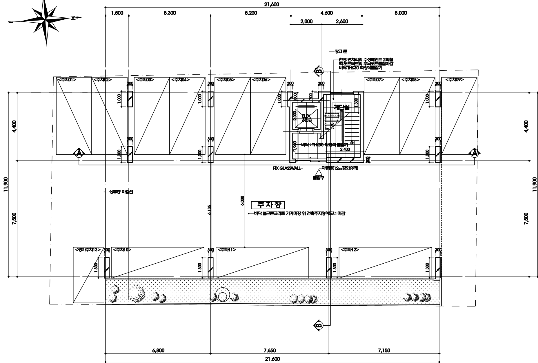
1층 평면도(변경후) Scale : 1/100
